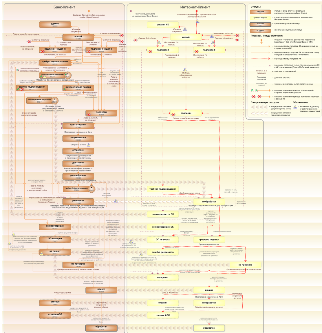
Рис. 5.175. Жизненный цикл заявлений на пополнение депозита
