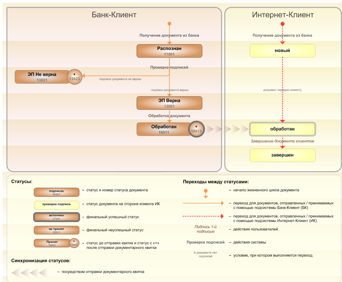
Рис. 5.154. Жизненный цикл произвольных документов из банка
