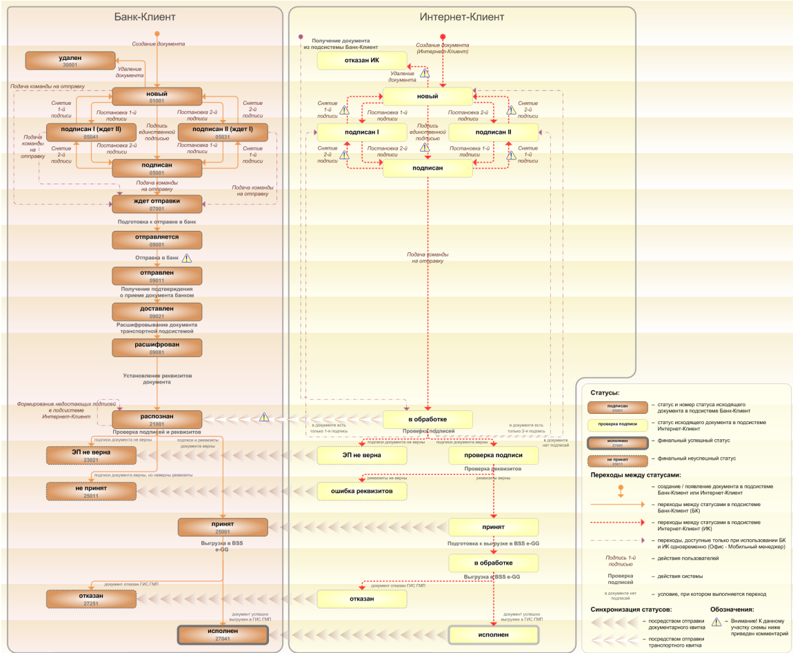
Рис. 5.159. Жизненный цикл запросов о начислениях
