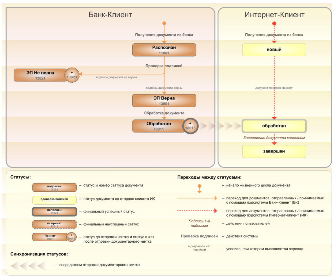
Рис. 5.141. Жизненный цикл уведомлений о зачислении средств на транзитный валютный счет
